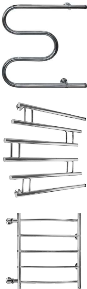
Полотенцесушитель, М-образный
